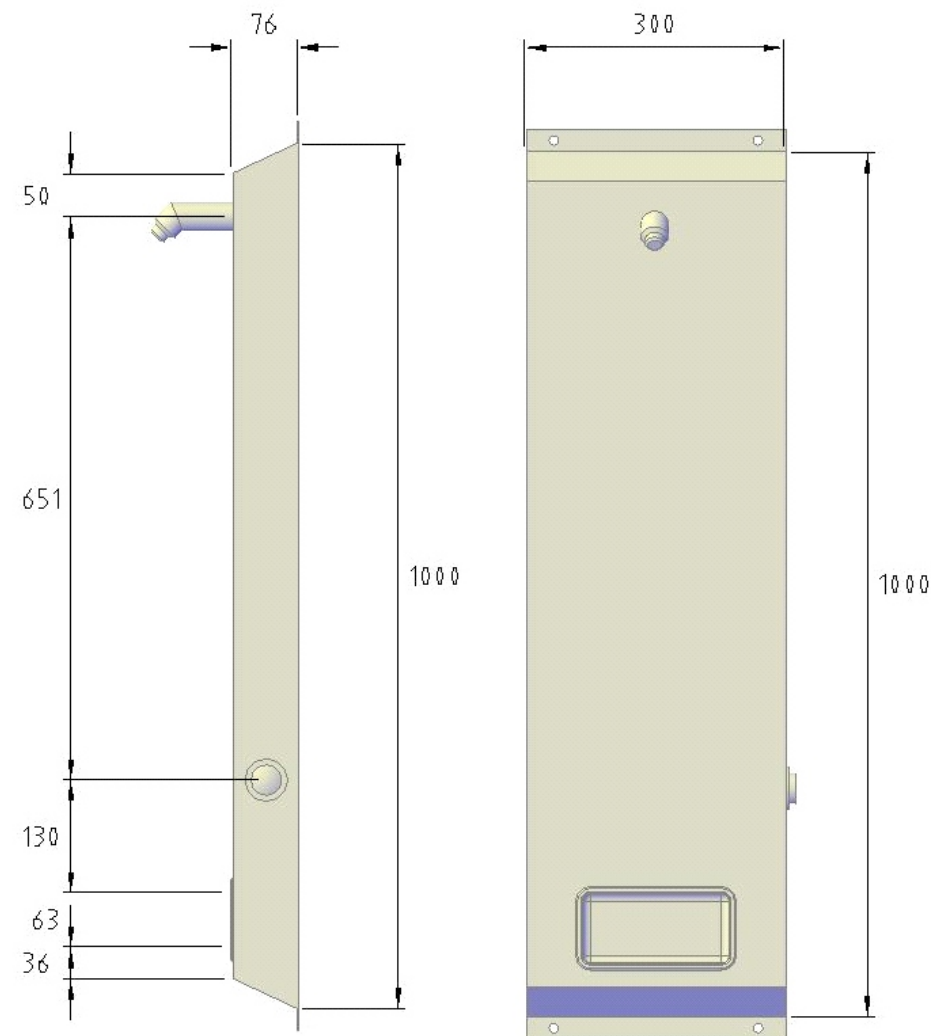
VISTA LATERAL
